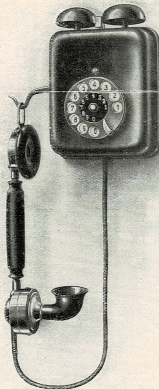
„Automat“-Wand-Fernsprechapparat in Metallgehäuse für vollautomatische Anlagen
