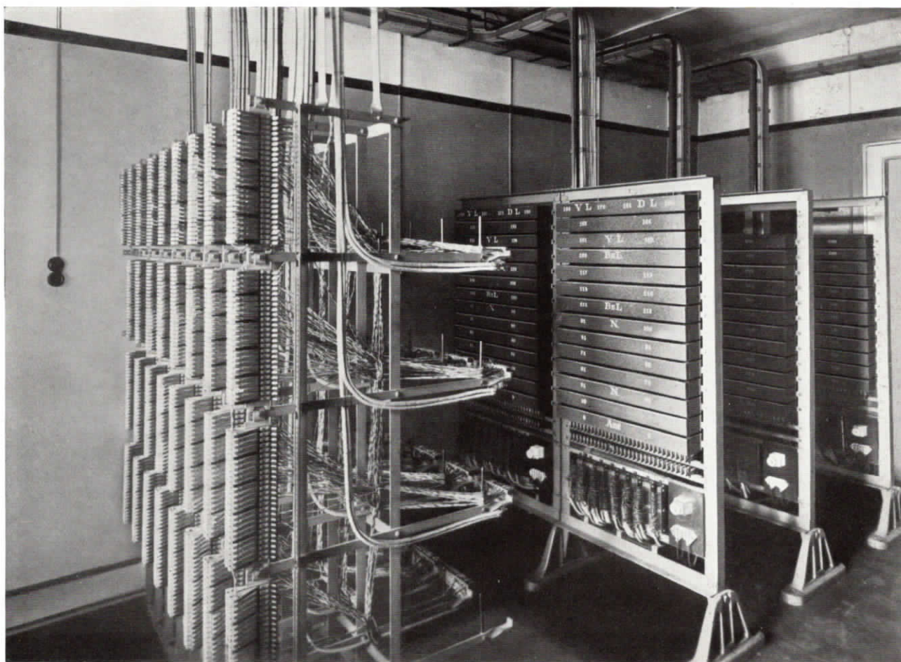
Abb. 4. Haupt- und Rangierverteiler sowie Relaisgestelle für die Zentralumschalter im Hauptbahnhof Chemnitz
