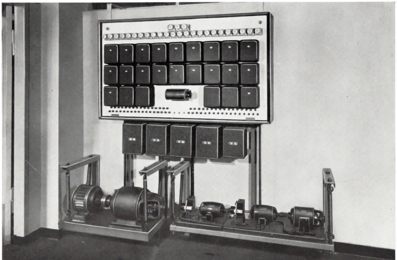
Abb. 5. Maschinenumformer zur Aufladung der Akkumulatorenbatterien, Signalmaschine für die Fernsprechanlage, Transformatoren- und Relais-Schalttafel für die Aufteilung des Personenrufes in 4 Gruppen, in der Allg. Ortskrankenkasse in Chemnitz
