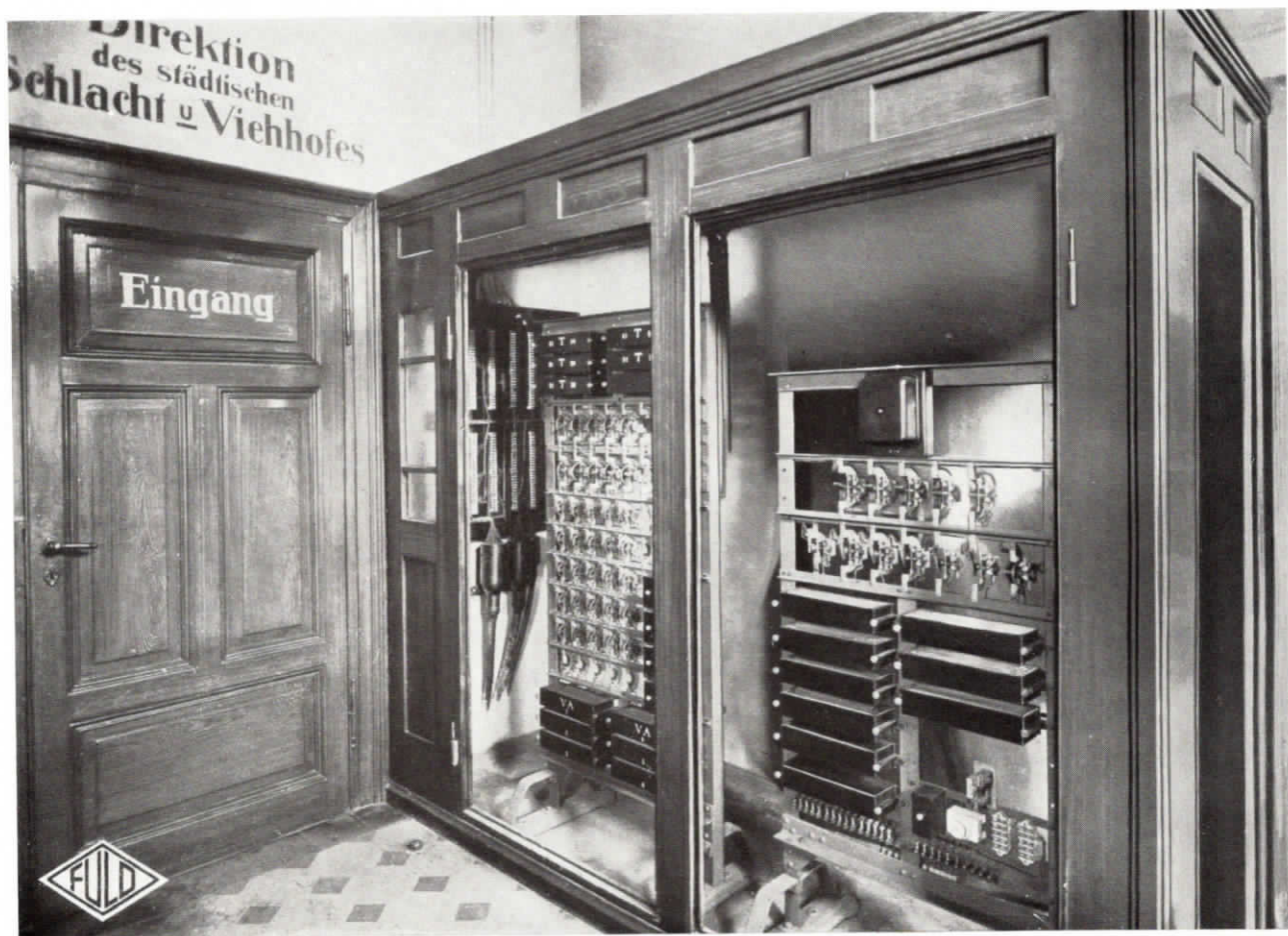
Abb. 6. Fuld-Fernsprech-Automatenzentrale im Städt. Schlacht- und Viehhof in Chemnitz
