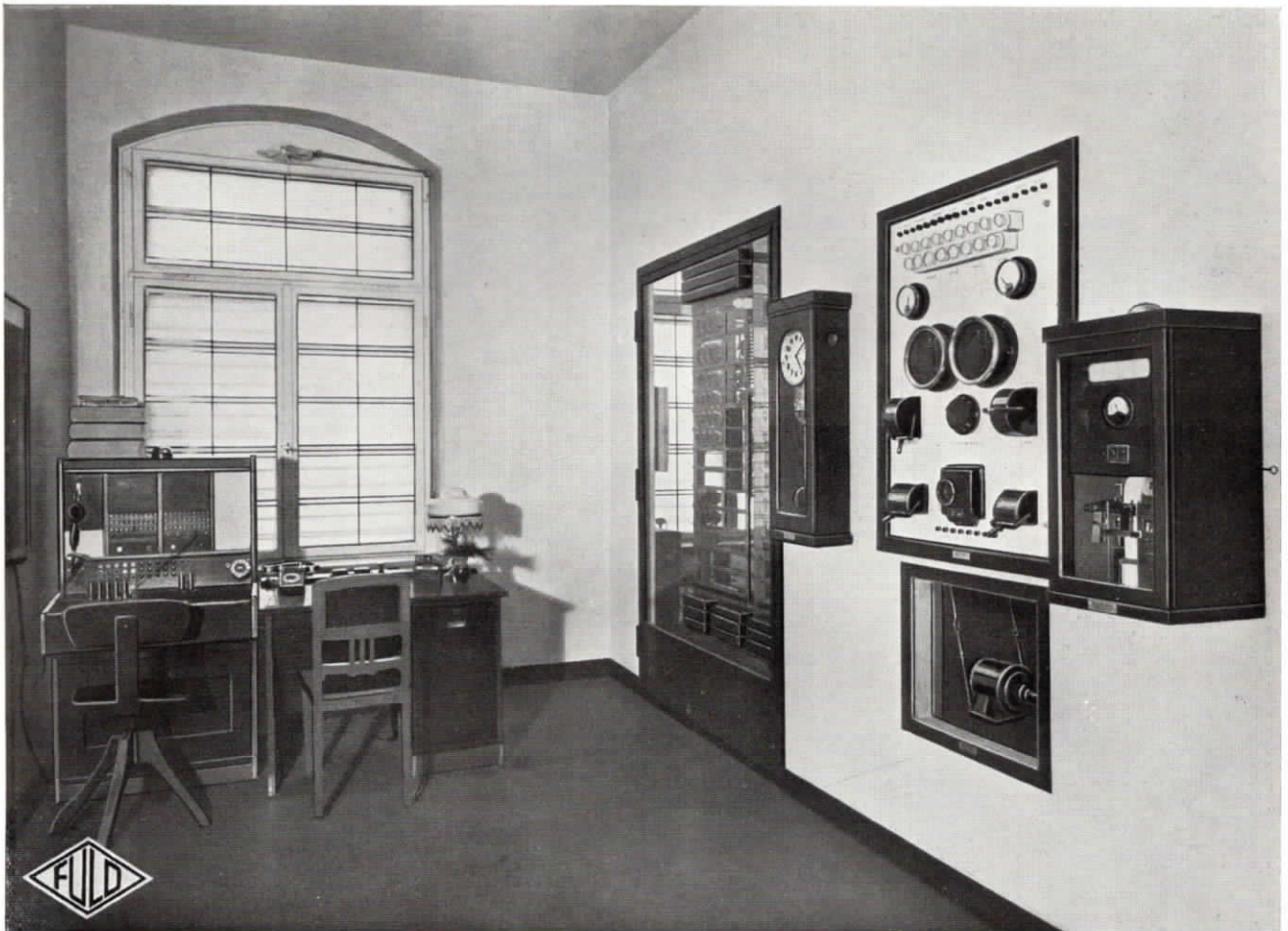
Abb. 37. Zentralenraum in der Gebrüder Becker Stoffhandschuhfabrik in Chemnitz mit Fuld-Fernsprech-Glühlampen-zentrale für 3 Amtsleitungen, einer Querverbindungsleitung und ca. 50 Nebenstellen
