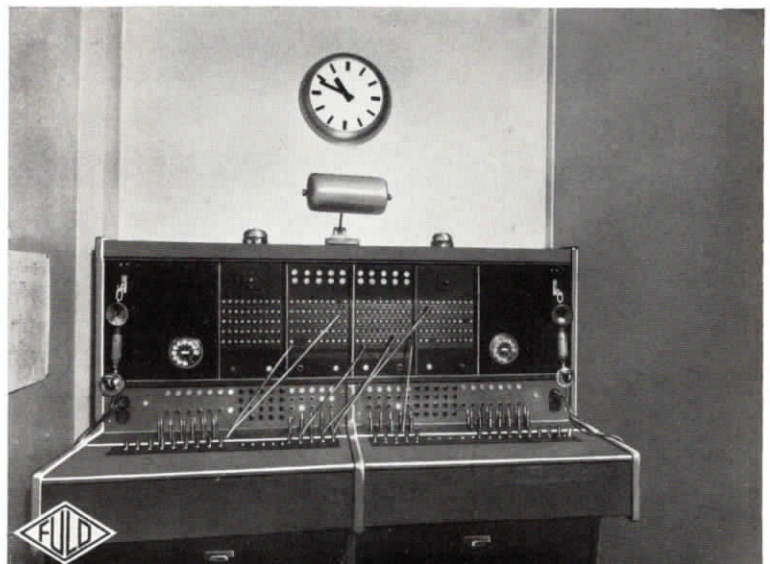
Abb. 21. Fuld-Fernsprechzentrale mit 2 Arbeitsplätzen für 10 Amtsleitungen und 200 Nebenstellen, sowie 15 Münzfernsprecher-Gegenkontrollampen, darüber elektr. Normalzeit-Nebenuhr im Hotel „Chemnitzer Hof“ in Chemnitz
