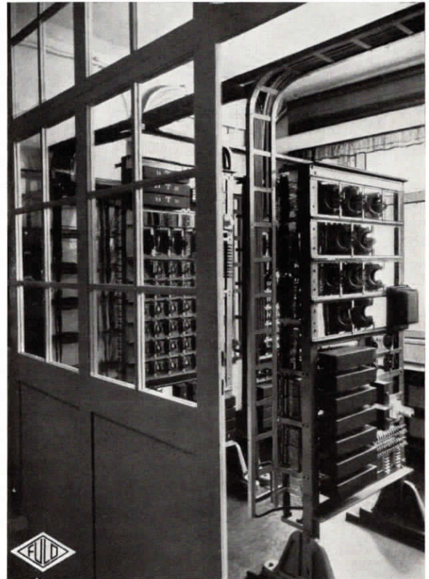
Abb. 14. Wähler- und Relaisgestelle für die halbautomatische Nebenstellenzentrale sowie für die vollautomatische Fuld-Hauszentrale im Werk I der Industrie-Werke A.-G. Plauen
