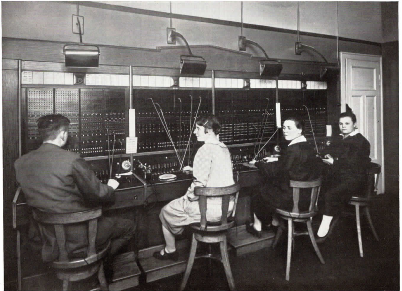
Abb. 2. Der Fuld-Fernsprechzentralumschalter mit 4 Arbeitsplätzen (Ortsschrank) im Hauptbahnhof Chemnitz
