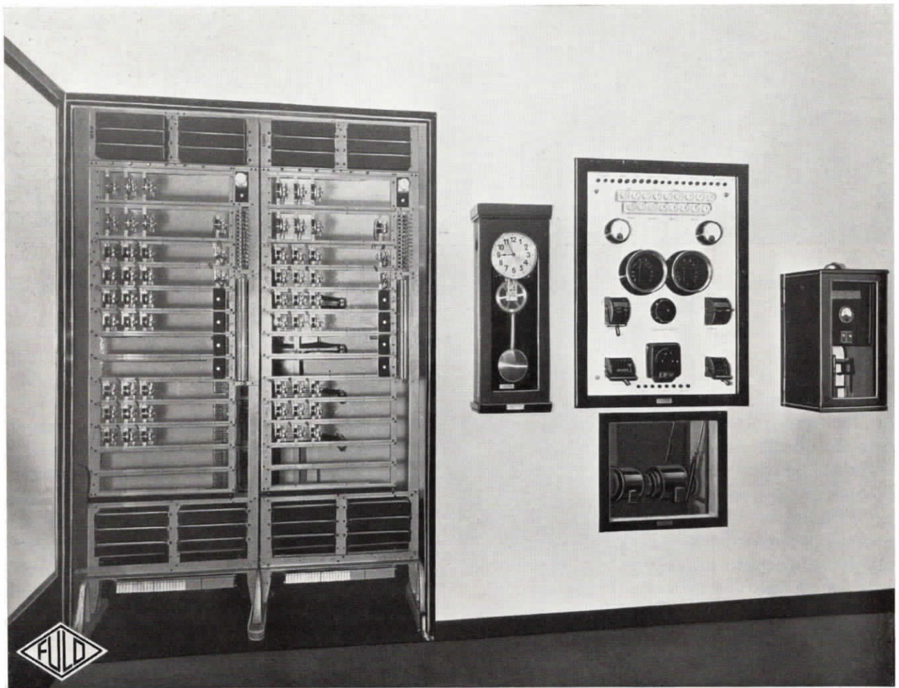
Abb. 38. Teilansicht des Zentralenraumes der Gebrüder Becker Stoffhandschuhfabrik in Chemnitz mit in einem Wandschrank eingebauter vollautomatischer Fuld-Fernsprechzentrale für 60 Teilnehmeranschlüsse, ferner elektrische Normalzeit-Hauptuhr mit Signaleinrichtung, Ladeschalttafel, Maschinenumformer zum Aufladen der Akkumulatorenbatterie sowie Wächterkontrollzentrale
