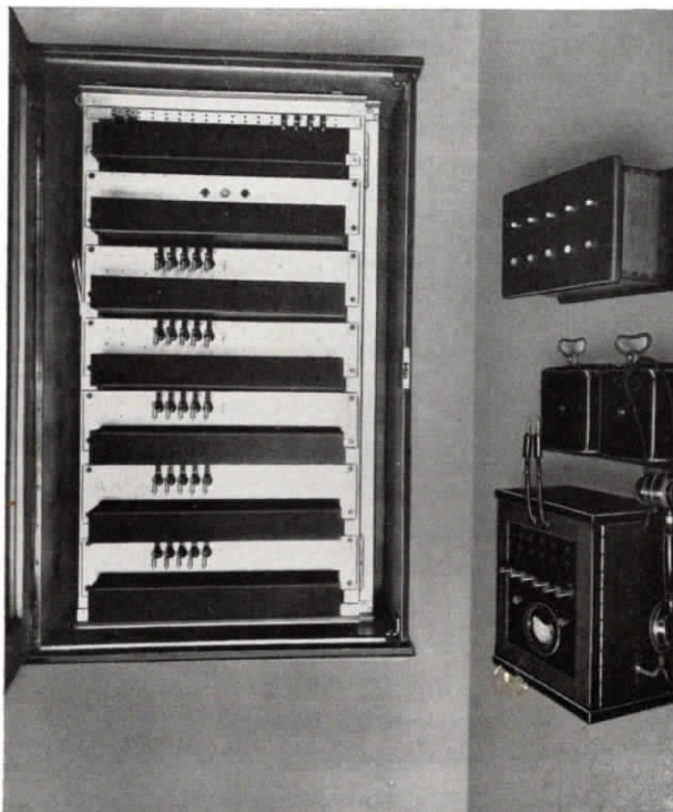
Abb. 2. Notruf-Empfangszentrale (mit Typendruckeinrichtung nach dem Dekadensystem) des Überfallkommandos im Polizei-Präsidium in Chemnitz
