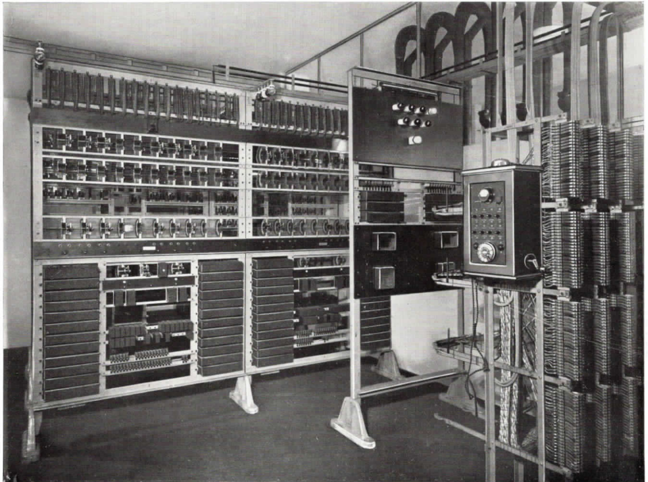
Abb. 3. Wähler und Relaisgestelle für die vollautomatische Fuld-Hauszentrale für 140 Teilnehmeranschlüsse nebst 3 Querverbindungsleitungen und für die halbautomatische Nebenstellenzentrale (Bild 2), ferner Haupt- und Rangierverteiler in der Allg. Ortskrankenkasse in Chemnitz
