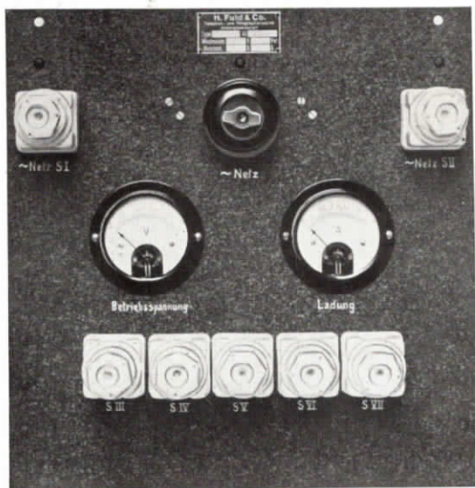
Abb. 2. Neues Fuld-Ladegerät (Vorderansicht)
