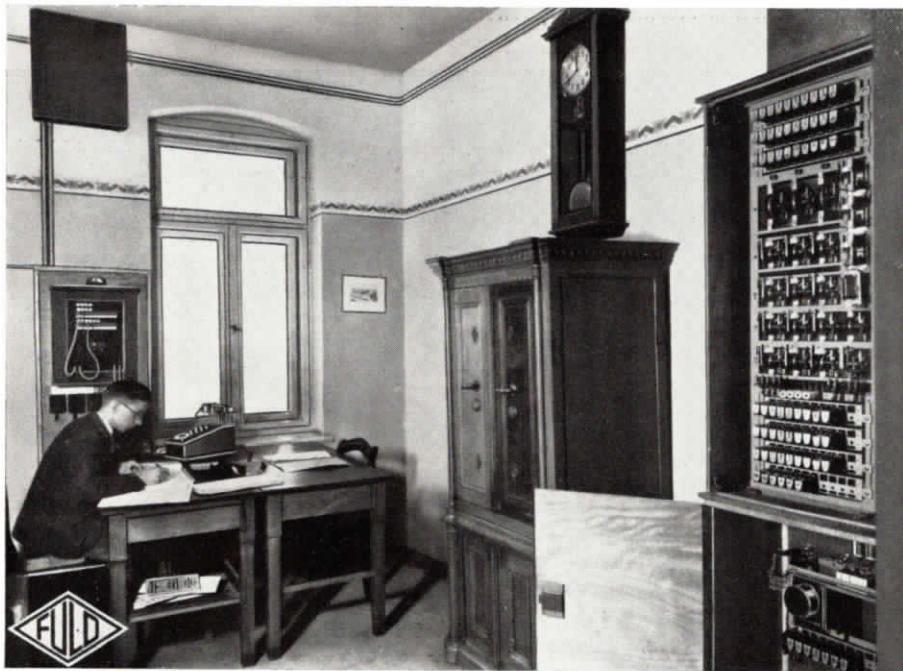
Abb. 21. Blick in den Zentralenraum im Verwaltungsgebäude des Bezirks-Konsum- und Sparvereins e. G. m. b. H. in Plauen. Die Fernmeldetechnische Anlage besteht a im Verwaltungsgebäude: aus einer Fuld-Fernsprech-Reihenanlage über 3 Amtsleitungen mit 14 Reihenapparaten und 4 Hausapparaten; dem internen Verkehr dient eine vollautomatische Fuld-Hauszentrale für 25 Teilnehmeranschlüsse und 2 Querverbindungen zur Unterzentrale im Warenhaus Bahnhofstraße, ferner aus einer elektr. Normalzeit-Uhrenanlage bestehend aus einer Hauptuhr und 12 Nebenuhren, b im Warenhaus Bahnhofstraße aus einer vollautomatischen Hauszentrale für 25 Teilnehmeranschlüsse mit 2 Querverbindungen zur Hauptzentrale im Verwaltungsgebäude
