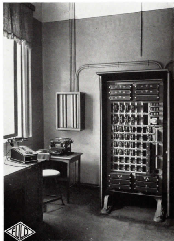
Abb. 19. Die Fuld-Fernsprechanlage in der Teppichfabrik Tefzet in Oelsnitz besteht aus 9 Reihenapparaten und 6 Hausapparaten, dem internen Verkehr dient eine vollautomatische Zentrale für 30 Teilnehmeranschlüsse
