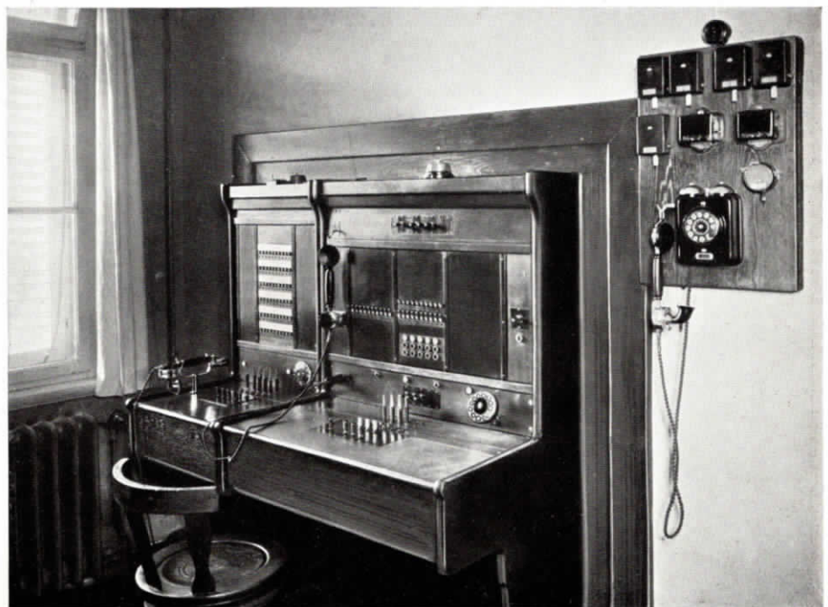
Abb. 9. Fuld-Halbautomatenzentrale der Städt. Straßenbahnen, Chemnitz
