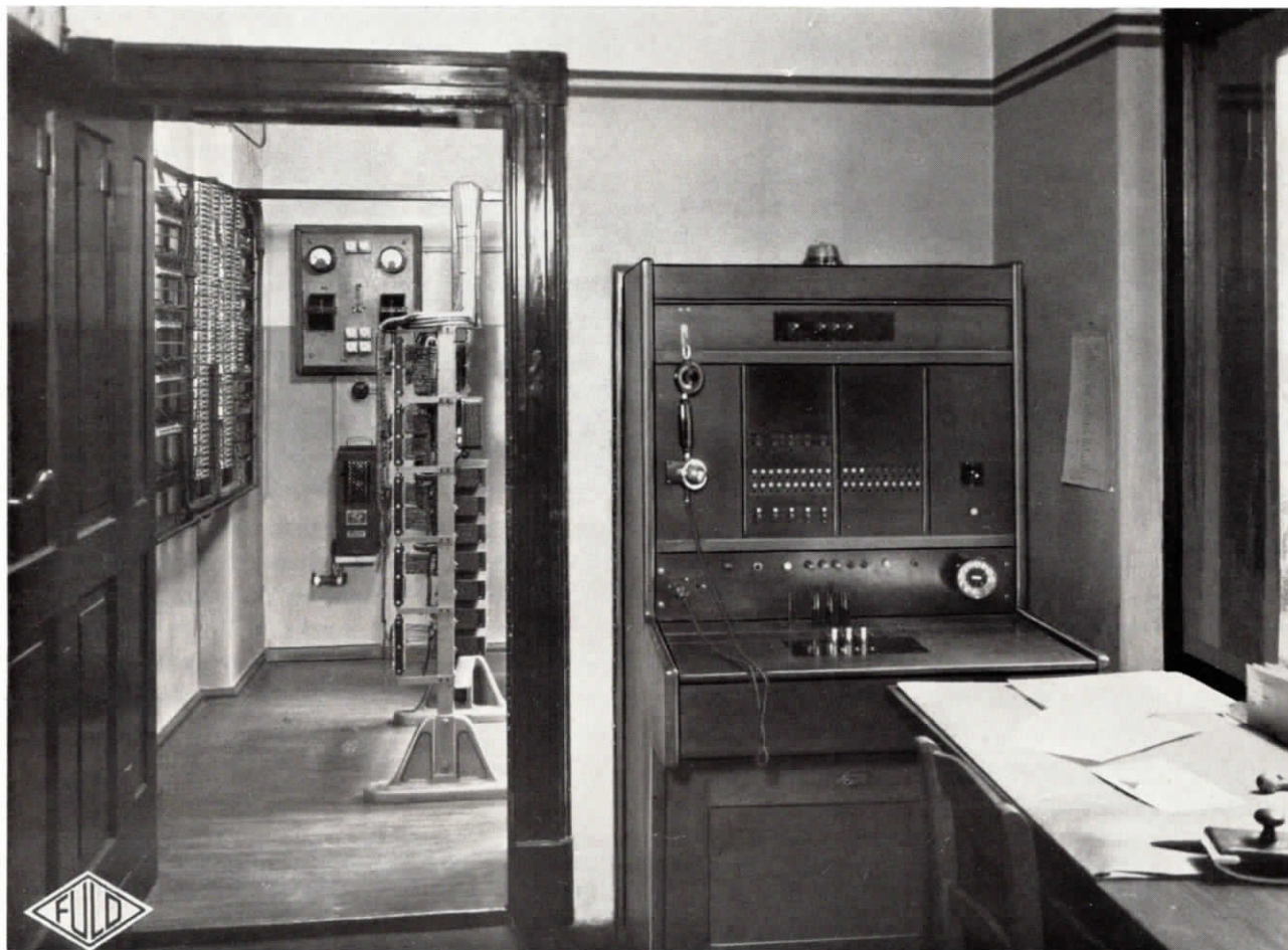
Abb. 2. Halbautomatische Fuld-Nebenstellenzentrale für 3 Amtsleitungen und 35 Nebenstellen; dem internen Verkehr dient eine vollautomatische Fuld-Hauszentrale für 40 Teilnehmeranschlüsse, in der Amtshauptmannschaft Plauen
