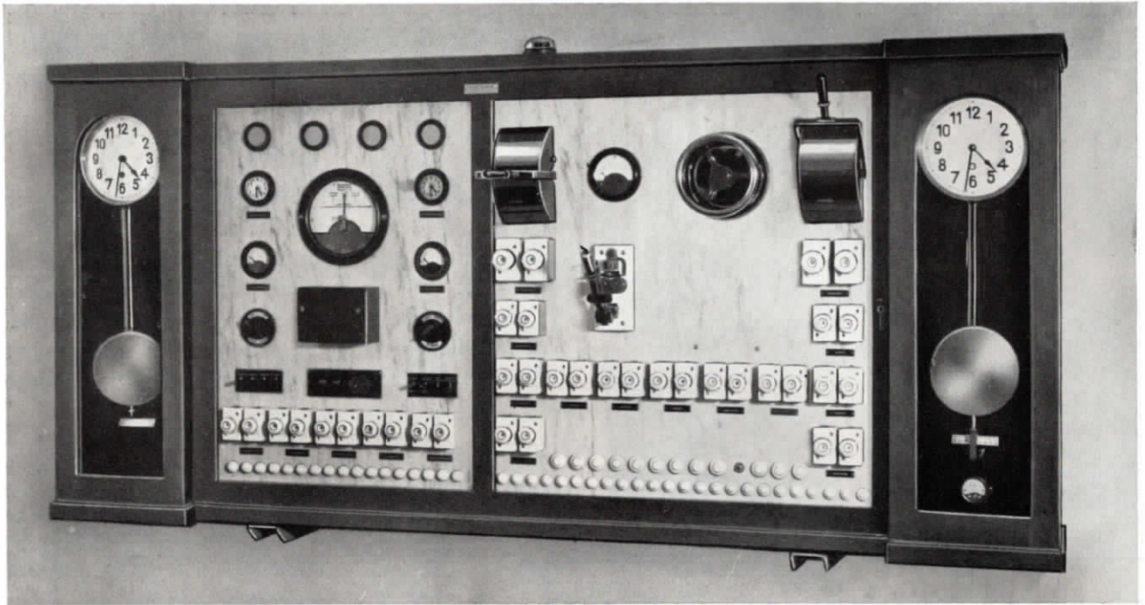
Abb. 4. Normalzeit-Uhrenzentrale, mit automatischer Umschaltung der Hauptuhr auf die Reserveuhr, für 2 Uhrenschleifen; kombiniert mit Ladeschalttafel für die gesamte Fernmeldeanlage, in der Allg. Ortskrankenkasse in Chemnitz
