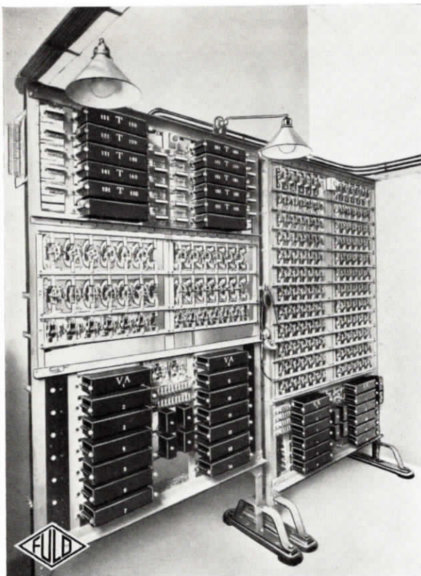
Abb. 14. Vollautomatische Fuld-Hauszentrale in der Dresdner Bank, Filiale Chemnitz
