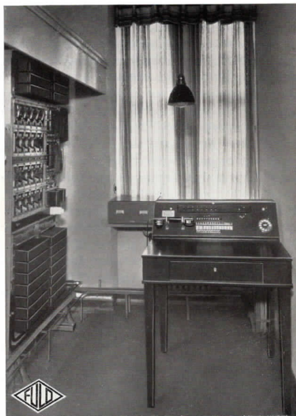
Abb. 34. Fernsprech-Zentralenraum der Aku-Verkaufskontor Glanzstoff Enka, in Chemnitz. Die Firma besitzt eine Fuld-Fernsprechanlage, bestehend aus einer halbautomatischen Nebenstellenzentrale in Pultform und einer vollautomatischen Hauszentrale für 30 Teilnehmeranschlüsse
