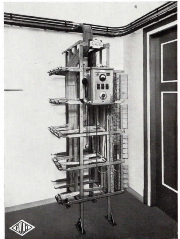
Abb. 15. Haupt- und Rangierverteiler der vollautomatischen Fuld-Hauszentrale in der Dresdner Bank, Filiale Chemnitz
