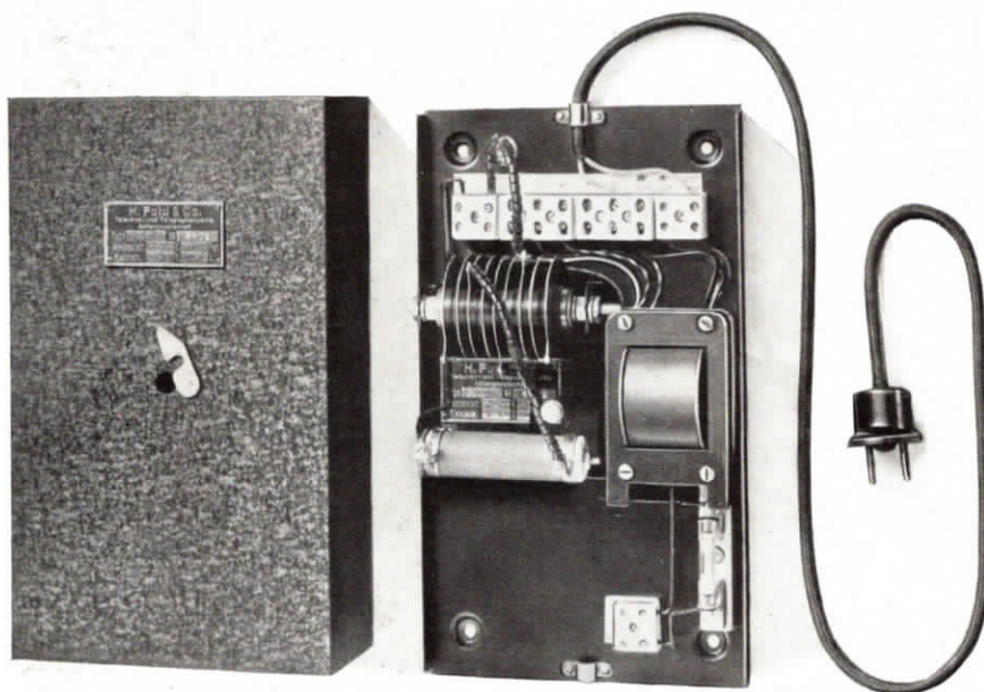
Abb. 4. Neues Fuld-Ladegerät für kleinsten Strombedarf
