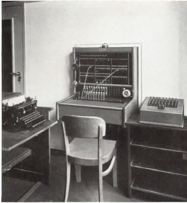
Abb. 2. Halbautomatische Fuld-Nebenstellenzentrale für 10 Amtsleitungen und 100 Nebenstellen. Rechts neben der Zentrale die Einschalttastatur für die Personen-Suchanlage mit Blinkleinrichtung zum Suchen von 25 Personen in der Allg. Ortskrankenkasse in Chemnitz
