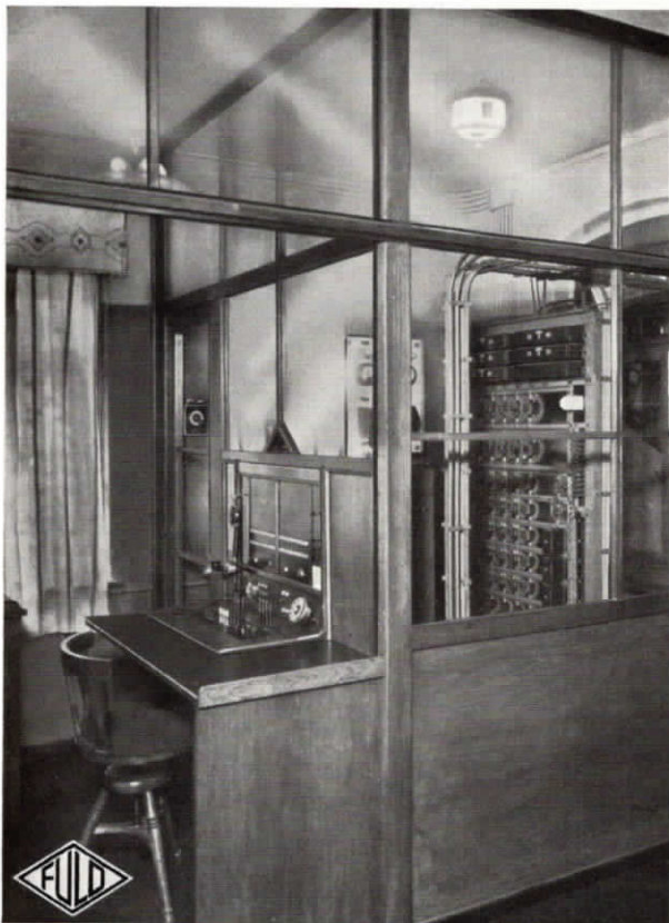
Abb. 27. Fuld-Fernsprech-Glühlampenzentrale für 3 Amtsleitungen und 40 Nebenstellen, sowie vollautomatische Fuld-Hauszentrale, ausgebaut für 40 Teilnehmeranschlüsse
