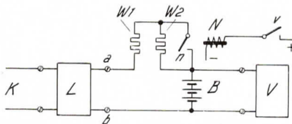
Abb. 1. Prinzipschaltung für das neue Fuld-Ladegerät
