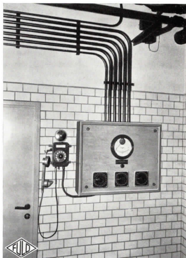
Abb. 15. Flur in der Badeanstalt für Frauen mit elektr. Fernthermometer im Vordergrund rechts, in der Allg. Ortskrankenkasse in Chemnitz
