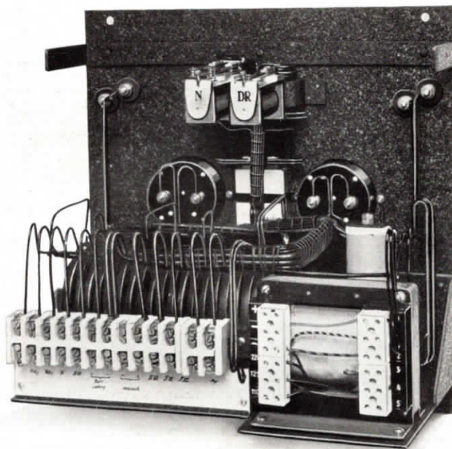
Abb. 3. Neues Fuld-Ladegerät (Rückansicht)
