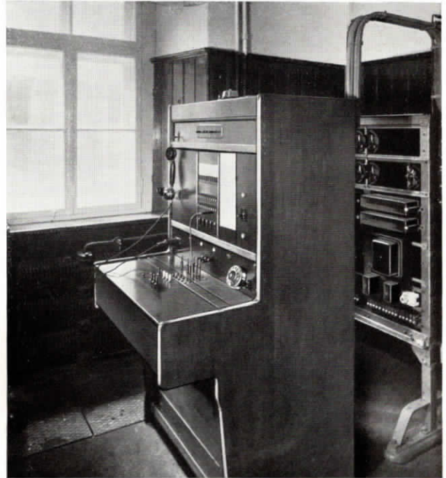
Abb. 8. Fuld-Halbautomat im Rathaus Burgstätt
