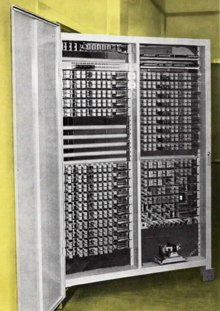
BILD 3 RELAISEINRICHTUNG EINER MAKLERANLAGE IN SCHRANKBAUWEISE
