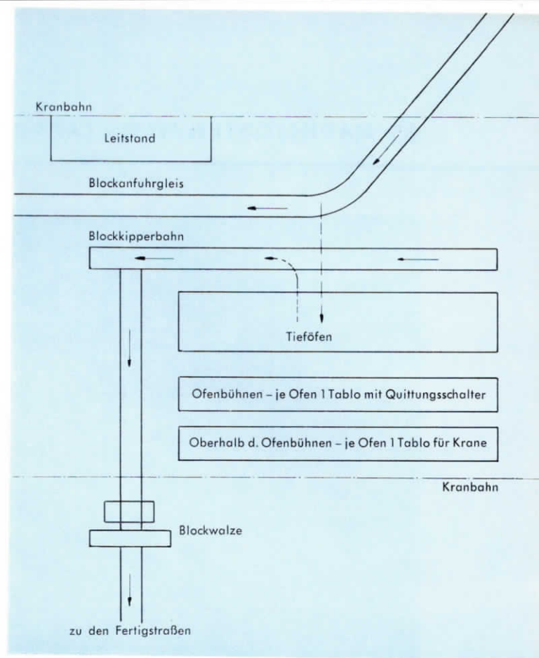
BILD 1 PRINZIPBILD DES ARBEITSABLAUFES IN DER TIEFOFENHALLE
