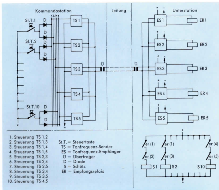
BILD 2 FERNWIRKANLAGE NACH DEM FREQUENZ-CODE-SYSTEM
