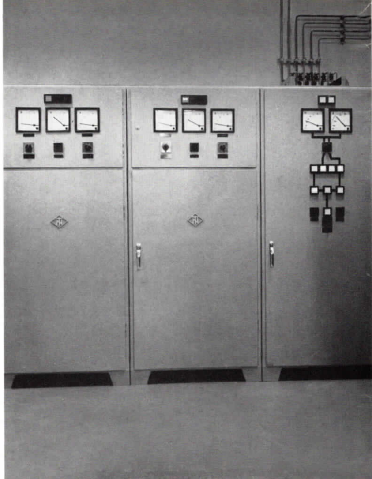
NETZSPEISEGERÄT 2 X 50 A MIT BATTERIEFELD
