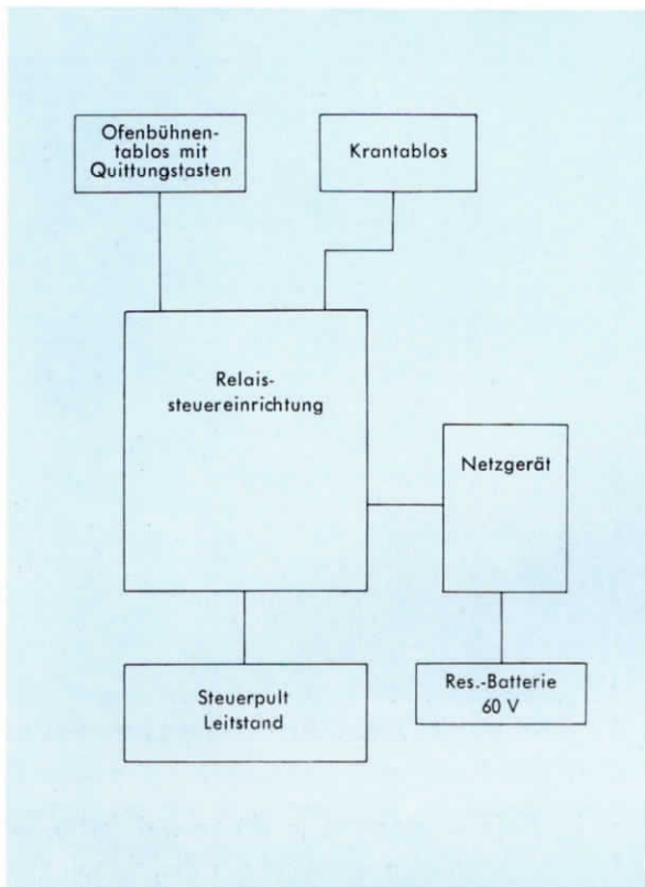
BILD 3 BLOCKSCHALTBILD DER TIEFOFENSIGNALANLAGE
