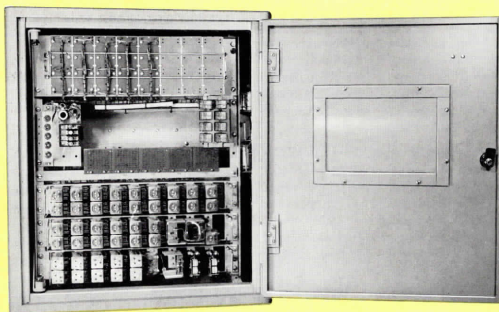
BILD 4 FERNWIRKANLAGE NACH DEM FREQUENZ-CODE-SYSTEM Übertragungsschrank, Kommandostation
