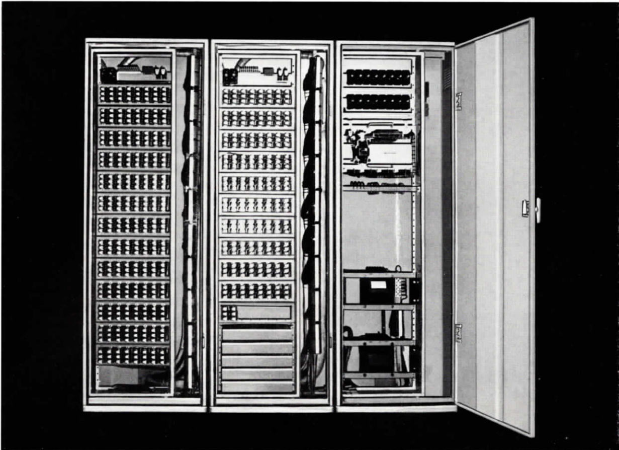
BILD 5 STEUEREINRICHTUNG DER SIGNALANLAGEN
