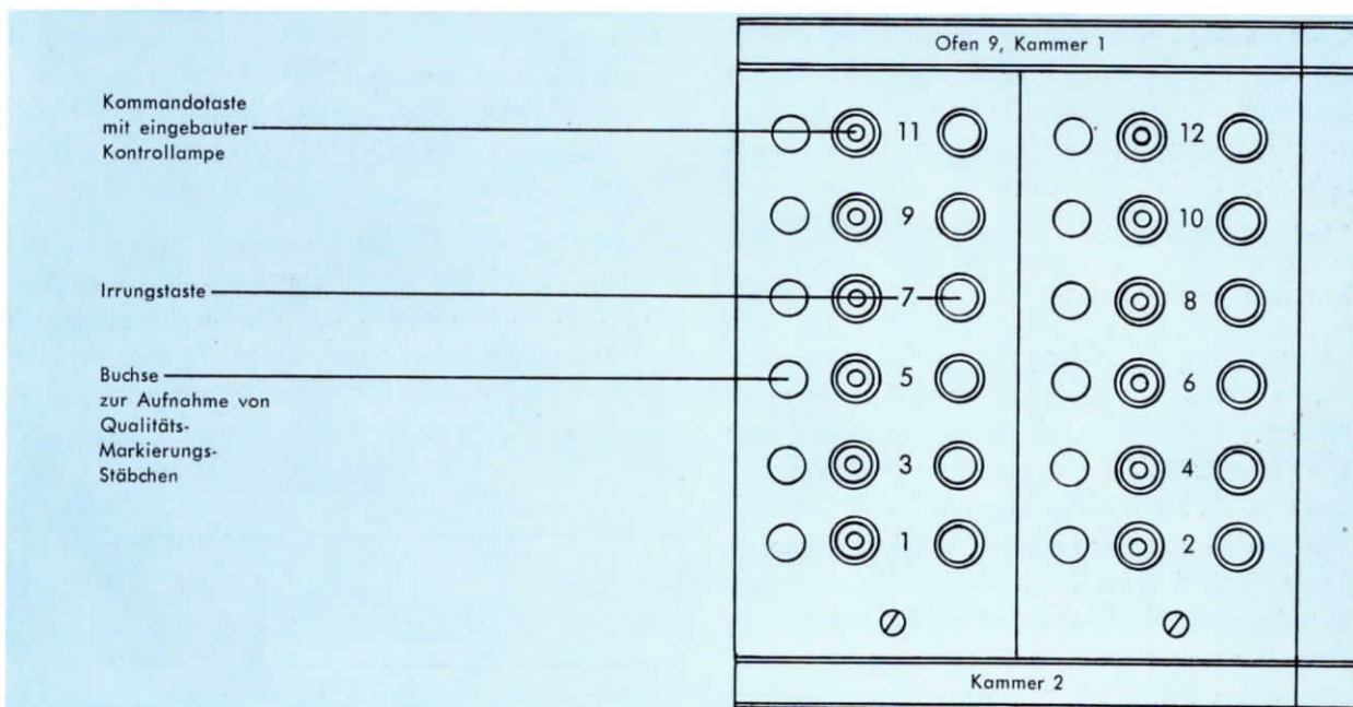
BILD 6 AUSSCHNITT AUS DER TASTENPLATTE DES STEUERPUOTES
