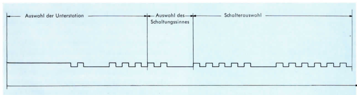
BILD 1 IMPULSTELEGRAMM EINER WÄHLERFERNSTEUERUNG
