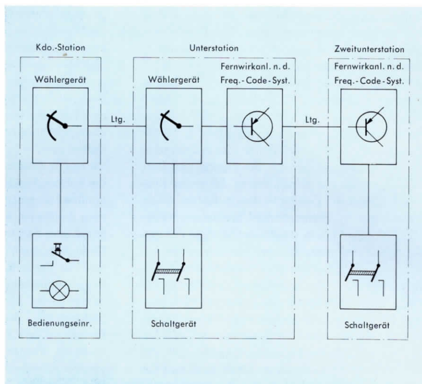
BILD 7 FERNWIRKANLAGE NACH DEM FREQUENZ-CODE-SYSTEM
