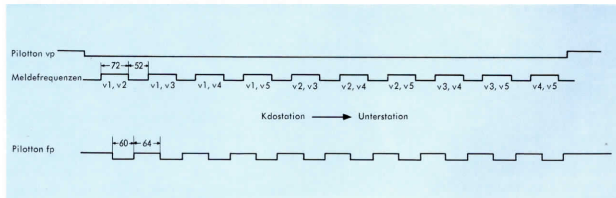
BILD 3 FERNWIRKANLAGE NACH DEM FREQUENZ-CODE-SYSTEM Impulsdiagramme von Steuerung, Schnellrückmeldung und Durchlaufender Signal-Meldung
