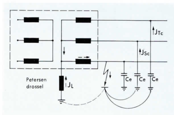
BILD 4 Stromverteilung im kompensierten Netz bei Erdschluß
