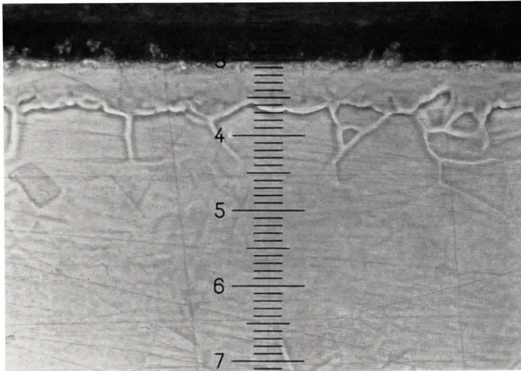
BILD 2 Querschliff durch die Oberflächenschicht eines vergoldeten Fe-Ni-Trägers nach der Diffusion Mikroskopische Vergrößerung = 500 : 1 T = 1173^{\circ} \text{K} z_{14} = 17,7 \mu d_{14} = 4,2 \mu \bar{x}_{14} = 13,5 \mu
