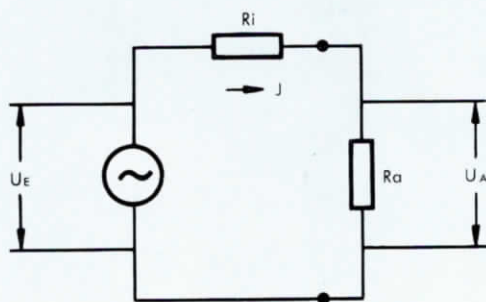
BILD 1 Ersatzschaltbild des Ausgangsrufkreises U_E = Spannung des Generators U_A = Ausgangs-Rufspannung am Widerstand R_a
