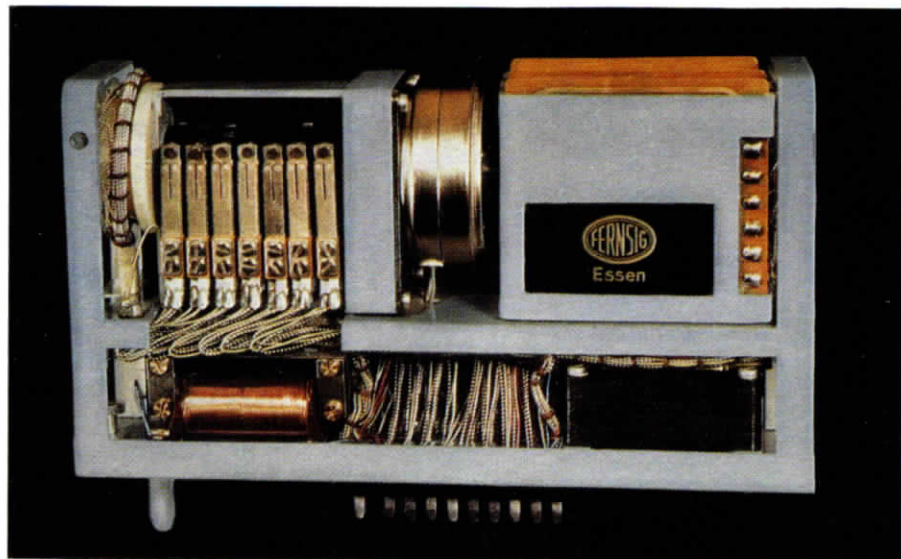
Ansicht der neuen Ruf-Signalmaschine
