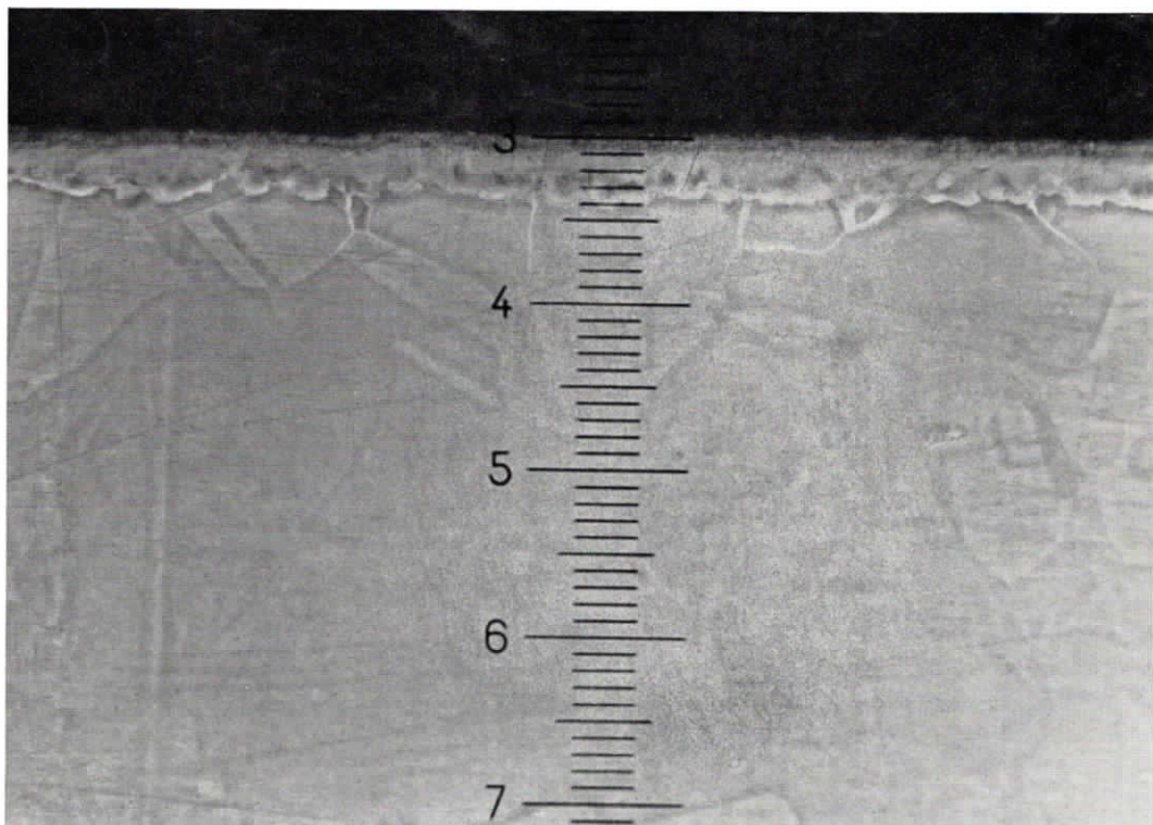
BILD 1 Querschliff durch die Oberflächenschicht eines vergoldeten Fe-Ni-Trägers nach der Diffusion Mikroskopische Vergrößerung = 500:1 T = 973^\circ K z_0 = 10,8 \mu d_0 = 6,0 \mu \bar{x}_0 = 4,8 \mu
