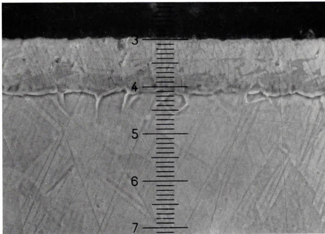
BILD 3 Querschliff durch die Oberflächenschicht eines vergoldeten Fe-Ni-Trägers nach der Diffusion Mikroskopische Vergrößerung = 500 : 1 T = 1273^{\circ} \text{K} z_{20} = 29,7 \mu d_{20} = 6,0 \mu \bar{x}_{20} = 23,7 \mu
