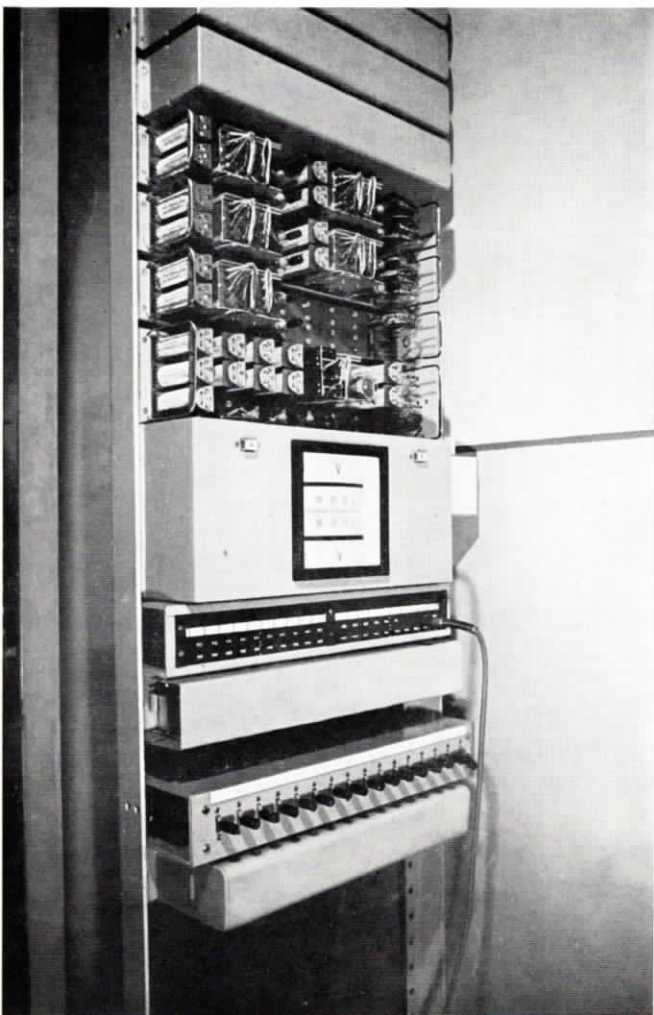
BILD 7 Knotenstelle mit Verstärker und Überwachung in der Verm. Ruhrort, Kästen geöffnet
