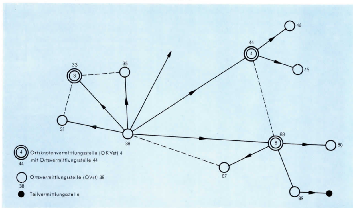
BILD 4 Von der OVSt 38 ausgehender Verkehr in einem Ortnetz (Ausschnitt)
